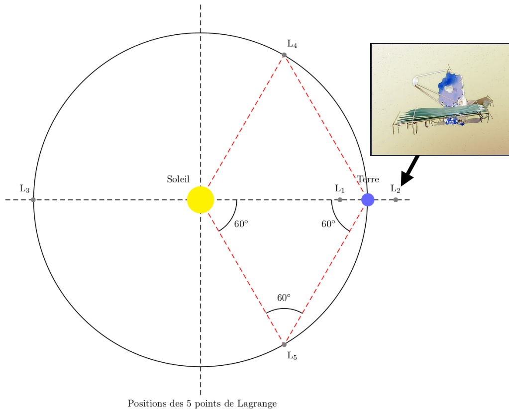
Positions des 5 points de Lagrange
